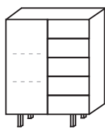
Senkki 90 1-ov./5 ltk (90 x 42 x 115)
